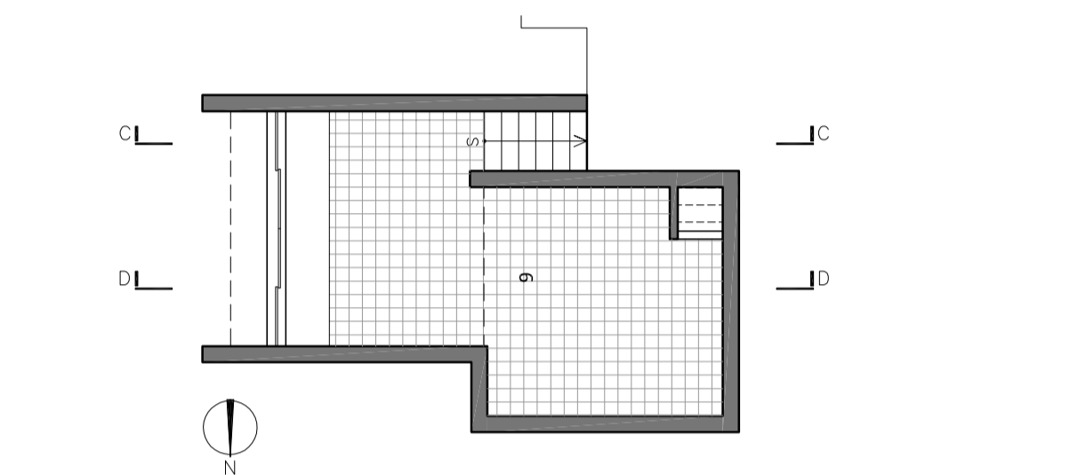
01 PLANTA PAV. INFERIOR ESC. 1/100
