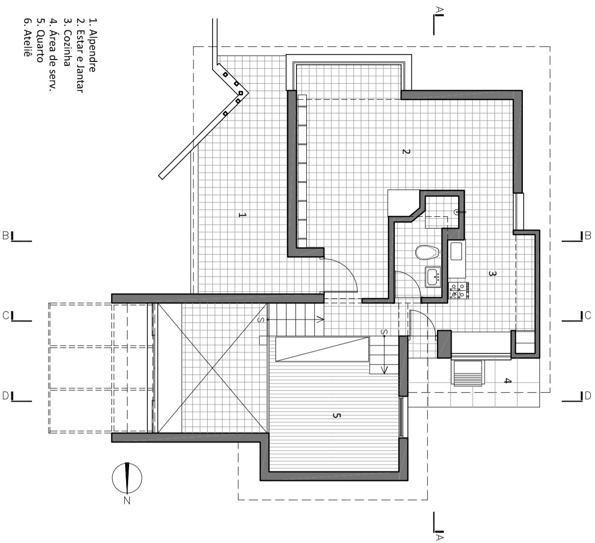
01 PLANTA PAV. TERREO ESC. 1/100
