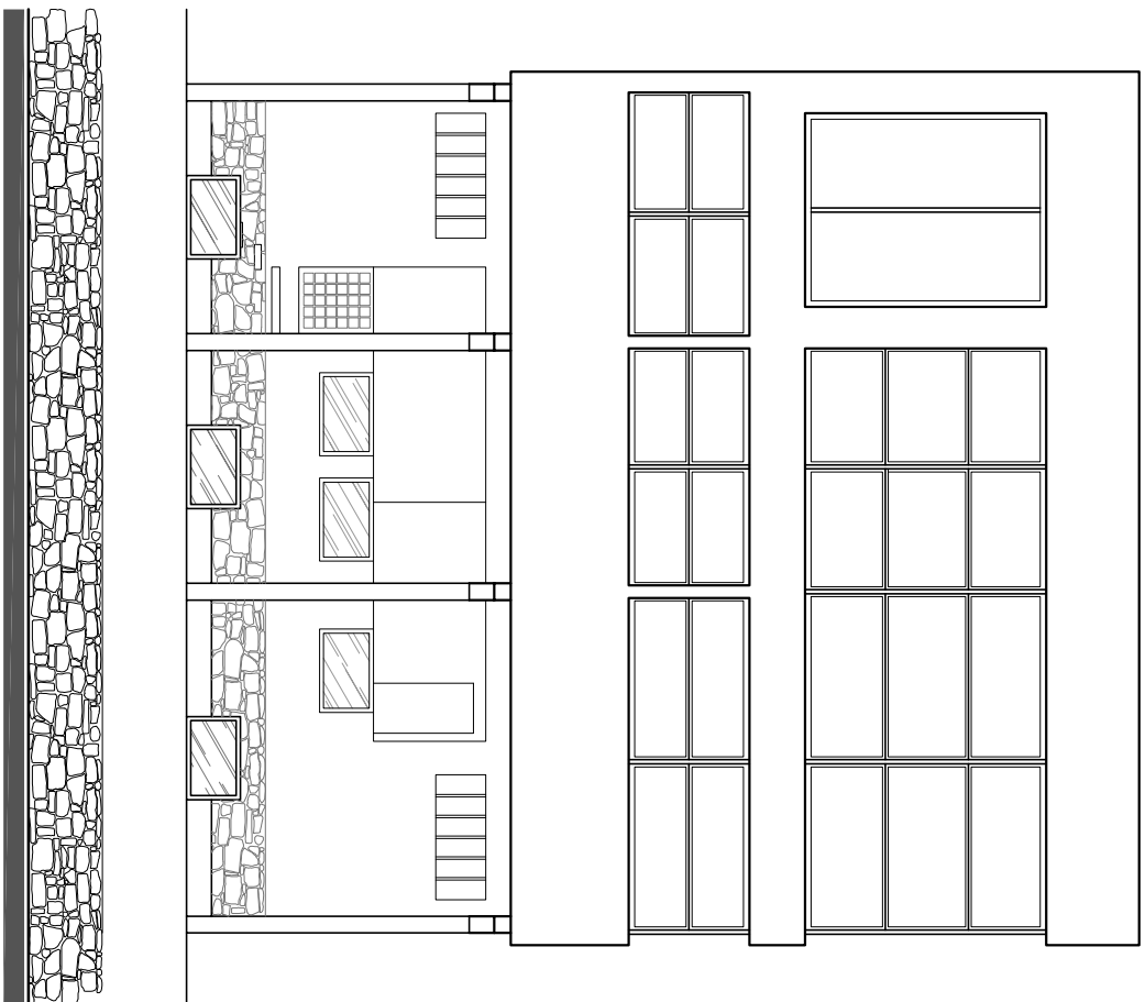
09 FACHADA SUL Esc. 1/100
