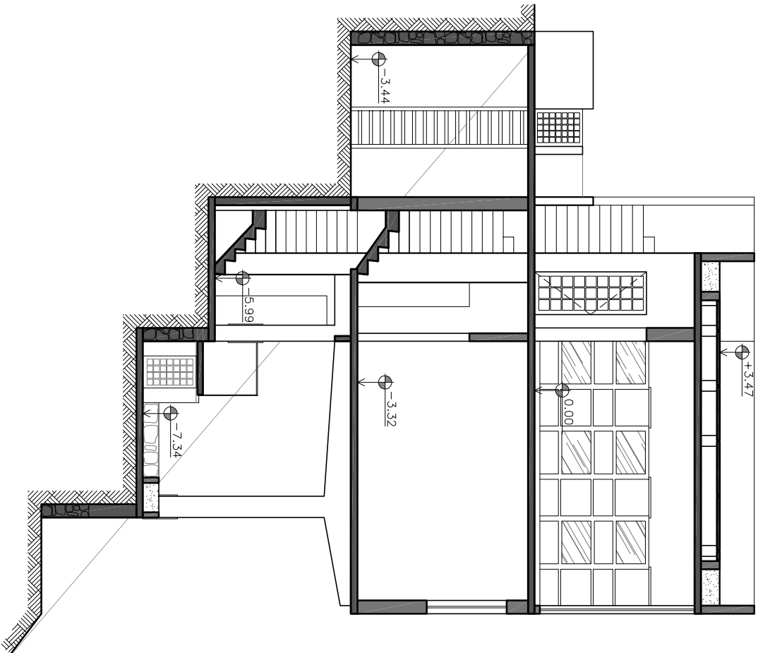
07 CORTE TRANSVERSAL B-B ESC. 1/100
