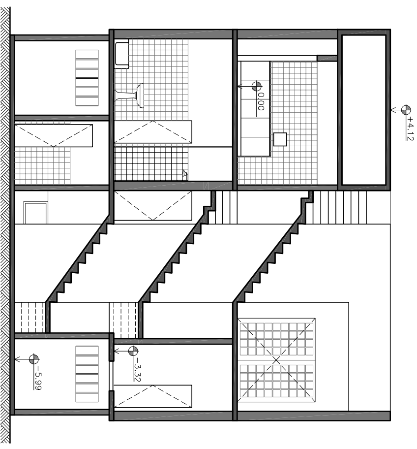
08 CORTE LONGITUDINAL C-C ESC. 1/100
