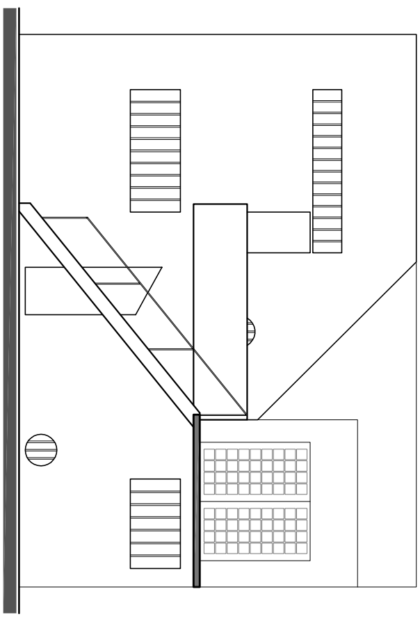
12 FACHADA NORTE ESC 1/100
