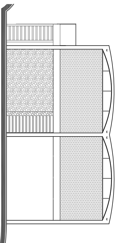
12 FACHADA NOROESTE ESC. 1/100
