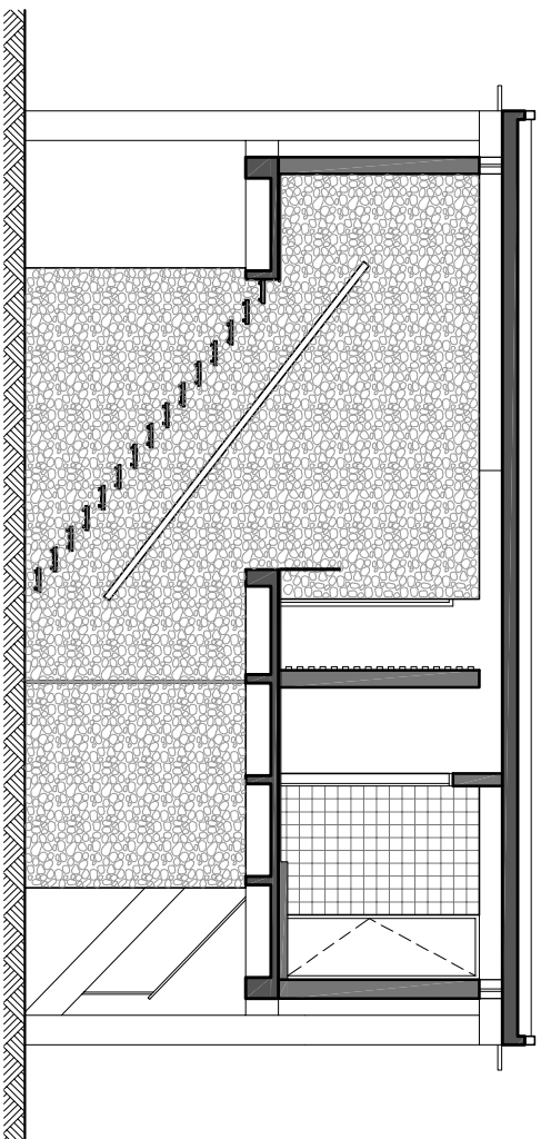
06 CORTE LONGITUDINAL A-A ESC. 1/100
