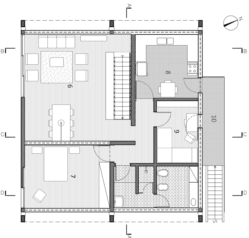
02 PLANTA PAVIMENTO SUPERIOR ESC 1/100
