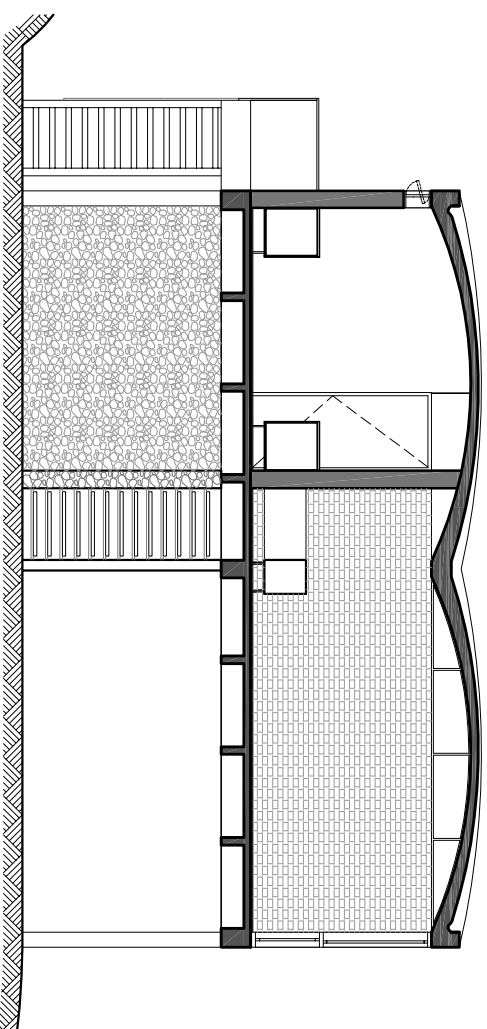
07 CORTE TRANSVERSAL B-B ESC. 1/100
